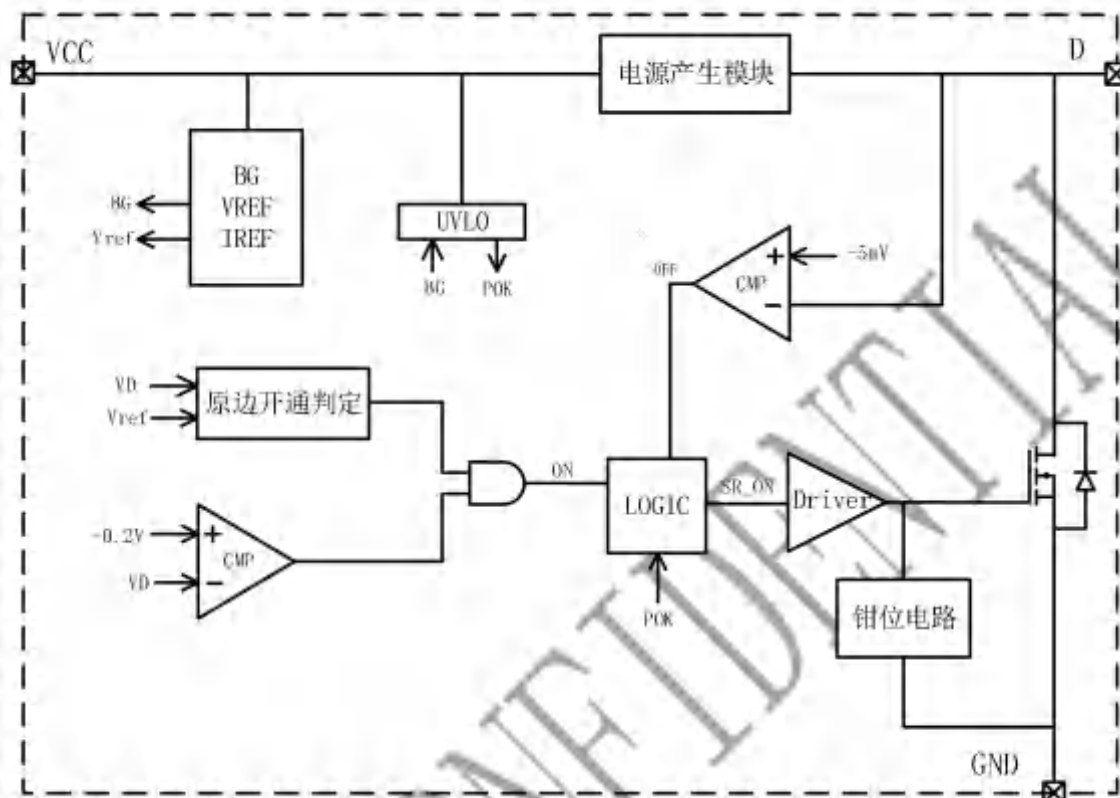
图3 LP3568G 内部框图
